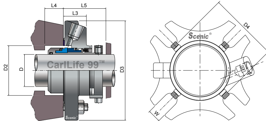
CarLife® 99™ - 公制标准尺寸
