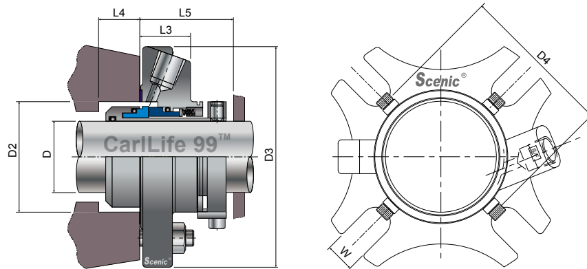
CarLife® 99™ - 英制加大 Enlarged Bore / 锥度 Tapered Bore 尺寸
