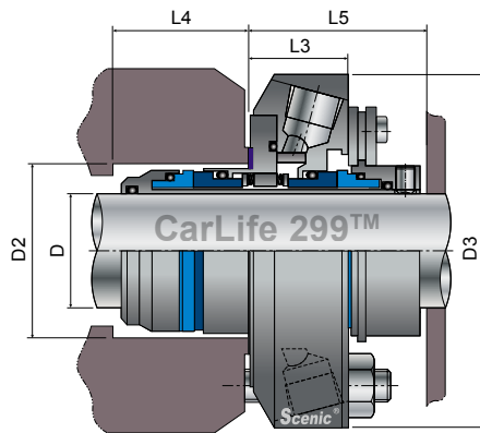
CarLife® 299™ - 公制标准尺寸
