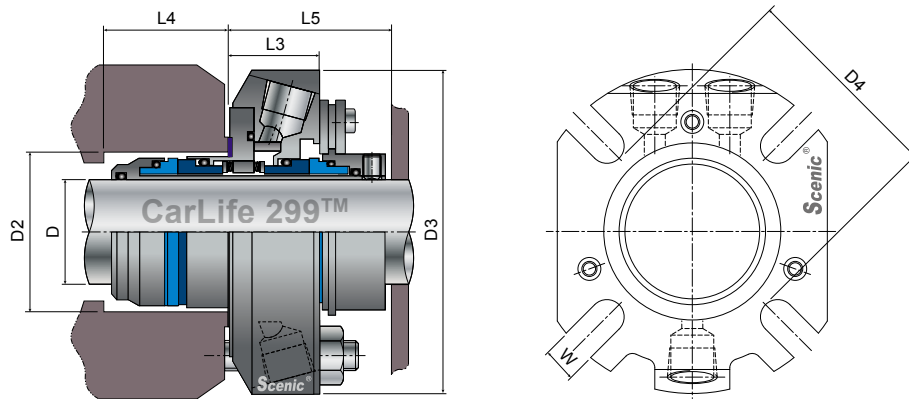
CarLife® 299™ - 英制加大 Enlarged Bore / 锥度 Tapered Bore 尺寸
